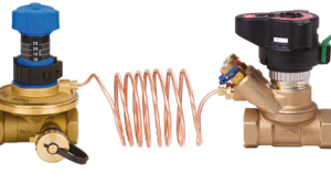
DPCV: ASV-PV+ASV-BD
