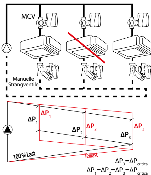
Abb. 11.2 Teillast – Umkehr-Rücklaufsystem
