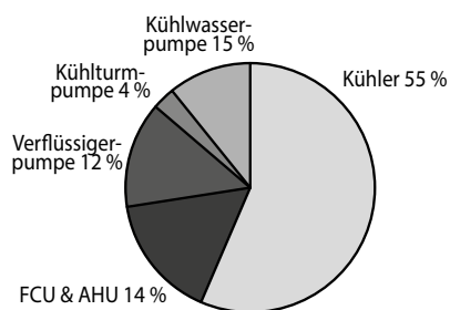
Aufteilung HVAC-Energieverbrauch
