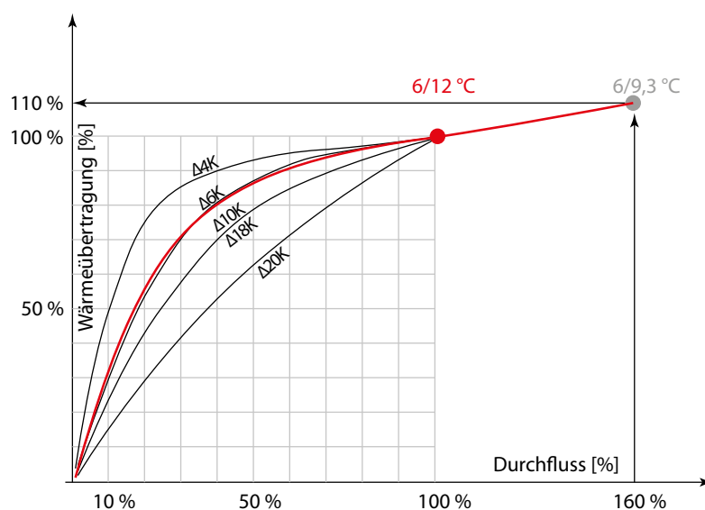
Abb. 12 Emissionskennlinie Endgerät
