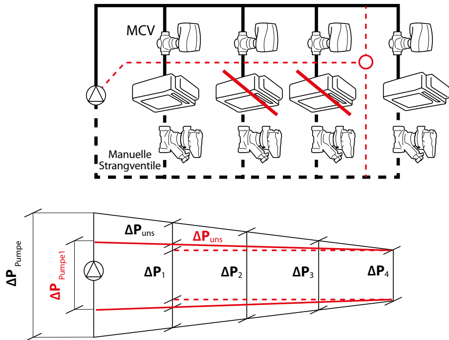
Abb. 14 Direktes System mit proportionaler Pumpenregelung
