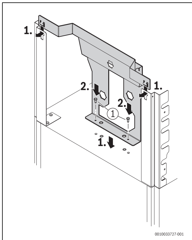
Bild 57 Basismodul (Zubehör CS 35) montieren – Schritt 2
