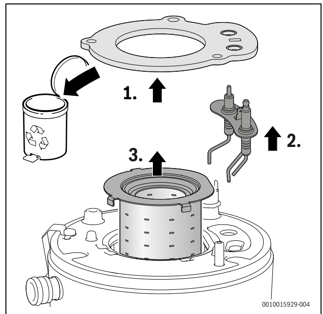
Bild 133 Brenner herausnehmen
