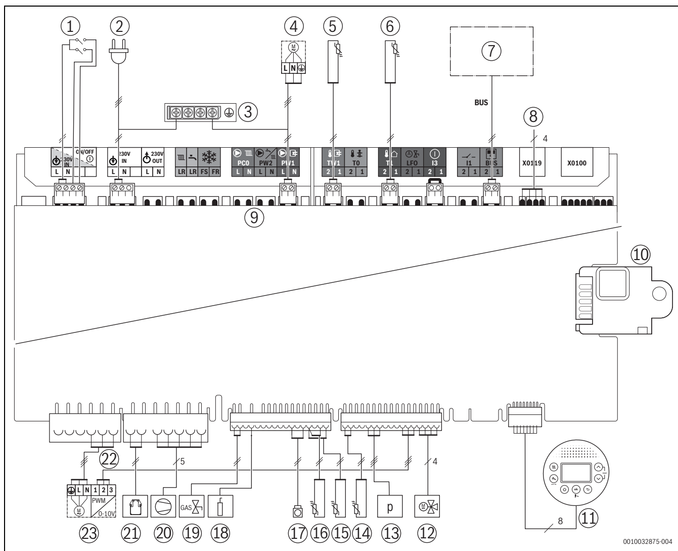
Bild 165 Elektrische Verdrahtung
