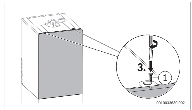
Bild 103 Vorderteil der Geräteverkleidung mit Schraube aus Lieferumfang sichern
