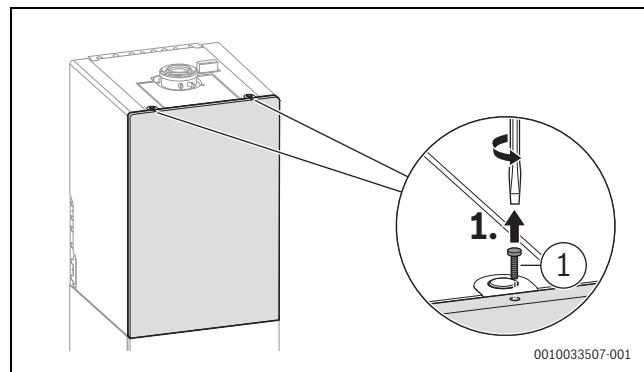
Bild 121 Sicherungsschraube lösen
