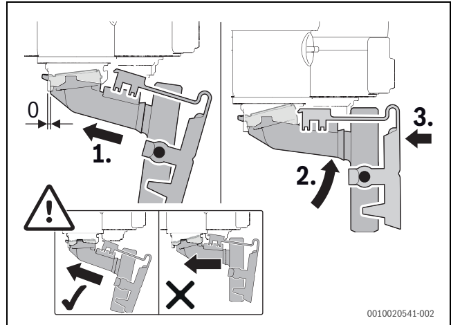
Bild 160 Kondensatsiphon einbauen
