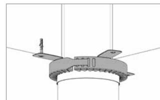
Massivdecke mit Dicke \geq 150 mm (siehe Einbauschritt 3)
