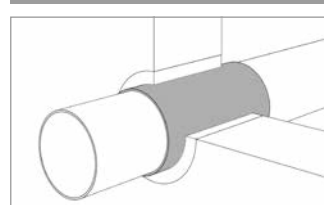
Ggf. Medienrohr mit einer handelsüblichen bis zu 5 mm starken Schalldämmung umwickeln. Restöffnung verschließen (siehe Seite 7).
