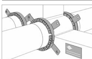
Die Manschetten können aneinander grenzen (Nullabstand).
