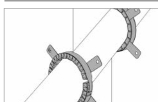
Rohrdurchführung schräg durch die Wand zugelassen.
