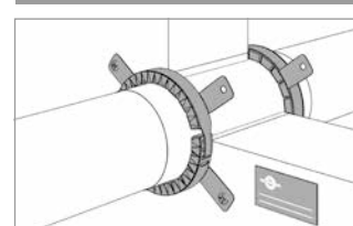
Manschetten mittels geeigneter Schrauben und Dübel mit der Wand verschrauben. Das Brandschutzschild ist zu beschriften und dauerhaft neben der Manschette zu befestigen.
