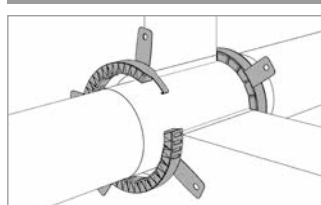
Manschette aufklappen um das Rohr legen und mittels Befestigungsbügeln verschließen.
