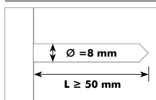
Position für Befestigungsbohrungen anzeichnen und anschließend Bohrungen setzen.
