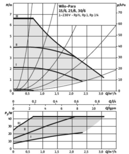
Konstant-Drehzahl
