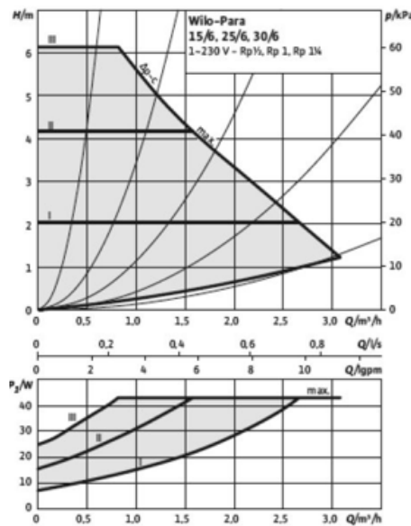
Differenzdruck konstant \Delta p_c
